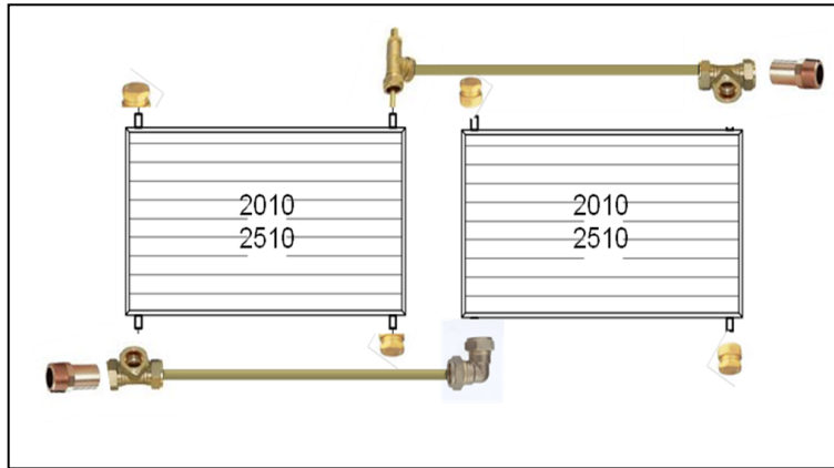
Abb. 1: Anschluss der Kollektoren, horizontal
