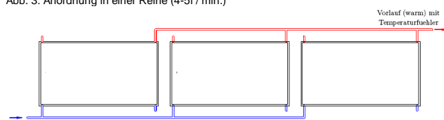
Abb. 6: Montage quer in einer Reihe nach Tichelmann (4-5l / min.)
