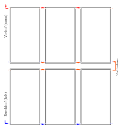
Abb. 4: Anordnung in zwei Reihen (4-5l / min.)
